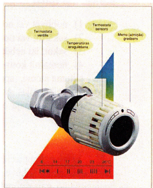
Attēls 3.4. Termostatiskais vārsts. Vārsts jāizslēdz, ja atver logu.
