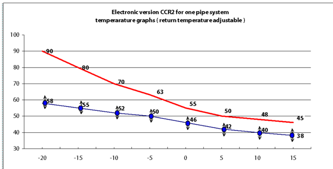
Attēls 4.2. Grafika vertikālā ass – siltumnesēja plūsmas temperatūra [°C], horizontālā ass – ārējais temperatūra [°C]. Sarkanā līkne – turpgaitas siltumnesēja plūsma, zilā līkne – atgaitas siltumnesēja plūsma.
